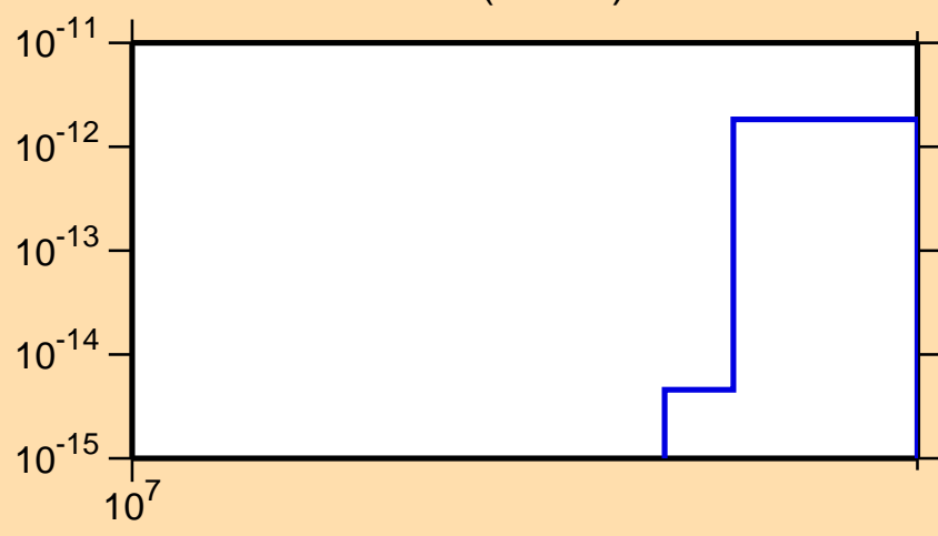
\sigma vs. E for ^{183}\text{Os} (mt 34)
