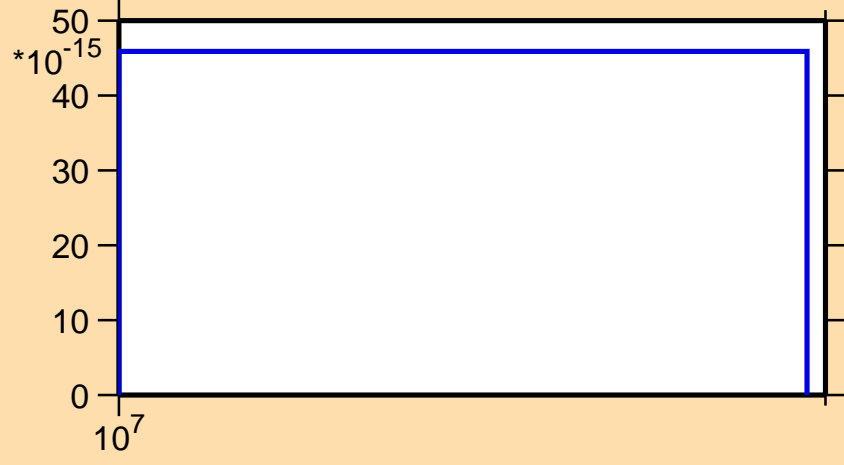
\sigma vs. E for ^{204}\text{Po} (mt 45)
