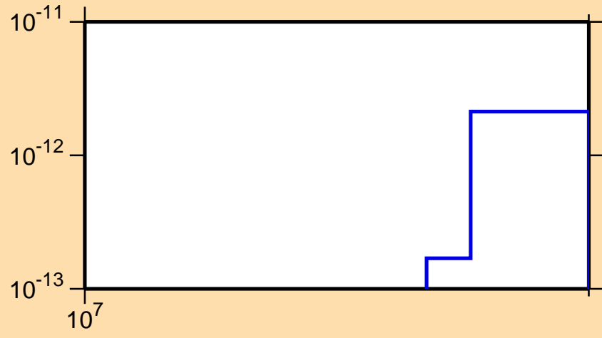
\sigma vs. E for ^{206}\text{Po} (mt 45)
