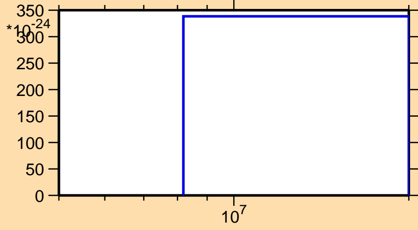
\sigma vs. E for ^{186}\text{Re}(\text{mt } 42)
