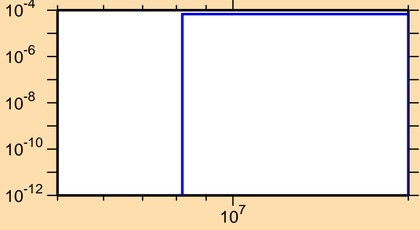
\sigma vs. E for ^{107}\text{Sb}(\text{mt } 45)
