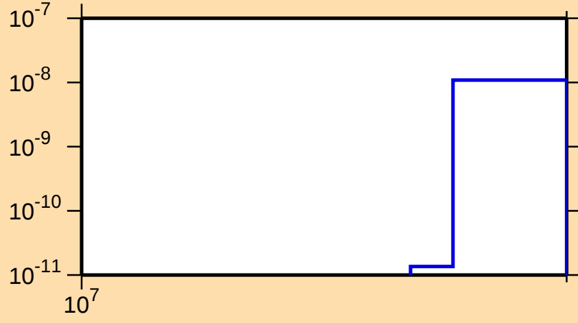
\sigma vs. E for ^{73}\text{Se}(\text{mt } 34)
