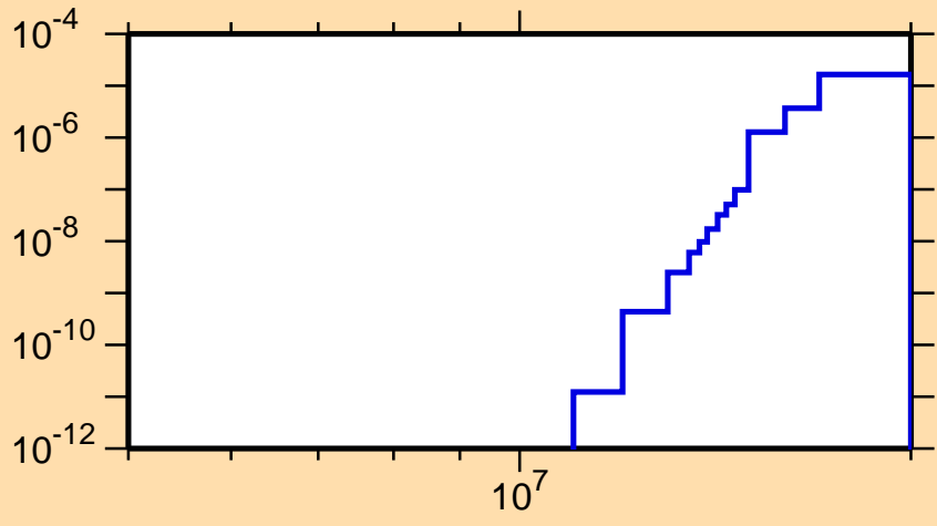
\sigma vs. E for ^{103}\text{Sn}(\text{mt } 45)
