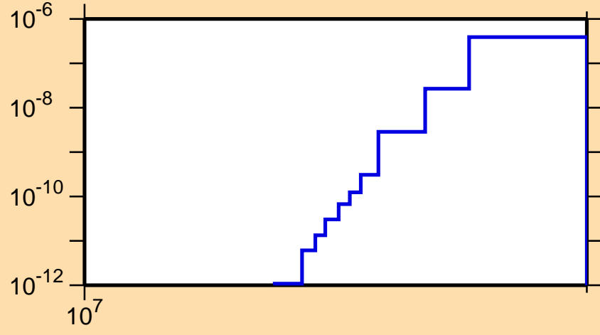
\sigma vs. E for ^{103}\text{Sn}(\text{mt } 34)
