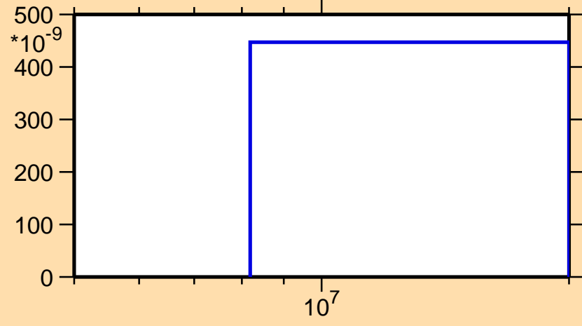
\sigma vs. E for ^{103}\text{Sn}(\text{mt } 45)
