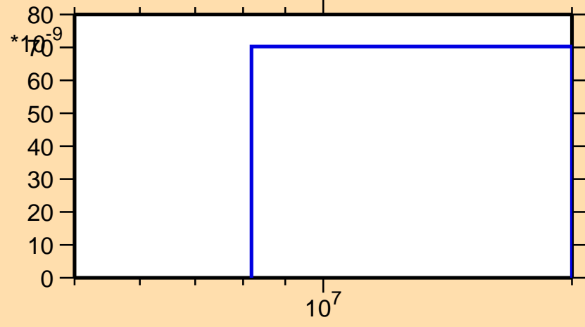
\sigma vs. E for ^{106}\text{Sn}(\text{mt } 45)
