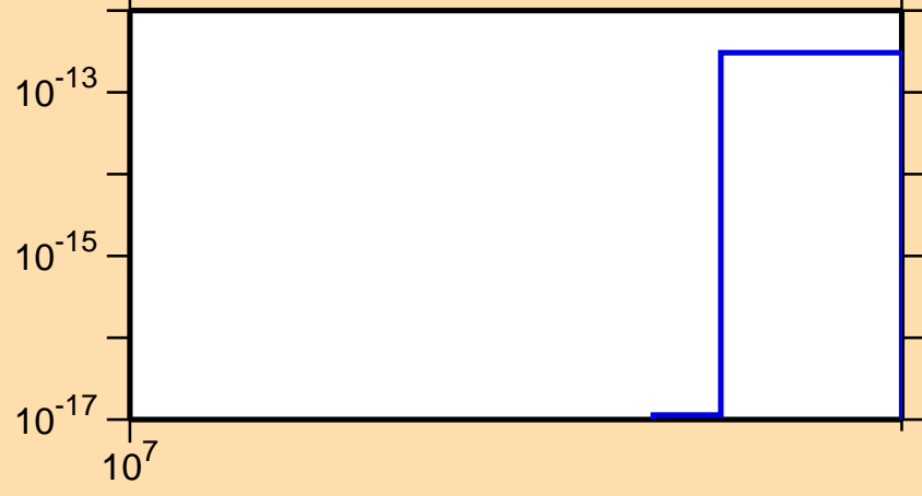
\sigma vs. E for ^{113}\text{Sn}(\text{mt } 34)
