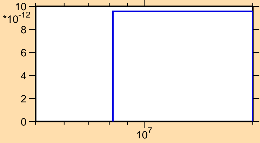
\sigma vs. E for ^{163}\text{Ta}(\text{mt } 34)
