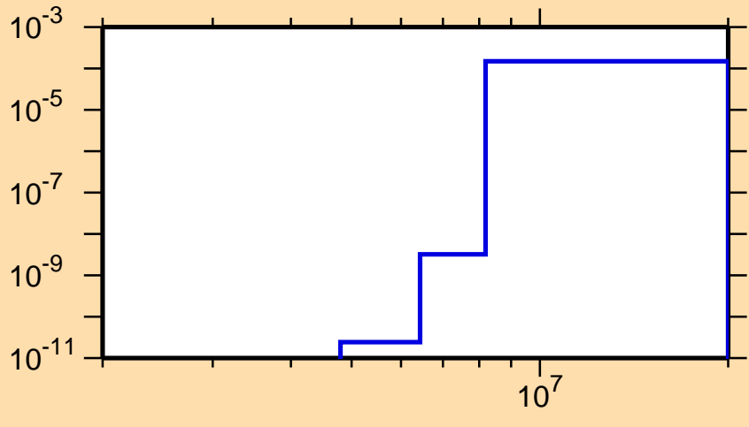
\sigma vs. E for ^{163}\text{Ta}(\text{mt } 45)
