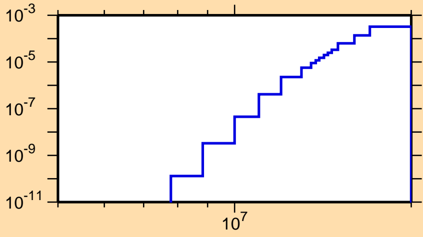
\sigma vs. E for ^{164}\text{Ta}(\text{mt } 45)
