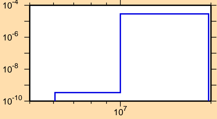
\sigma vs. E for ^{164}\text{Ta}(\text{mt } 45)
