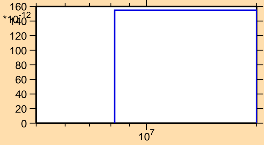
\sigma vs. E for ^{164}\text{Ta}(\text{mt } 34)
