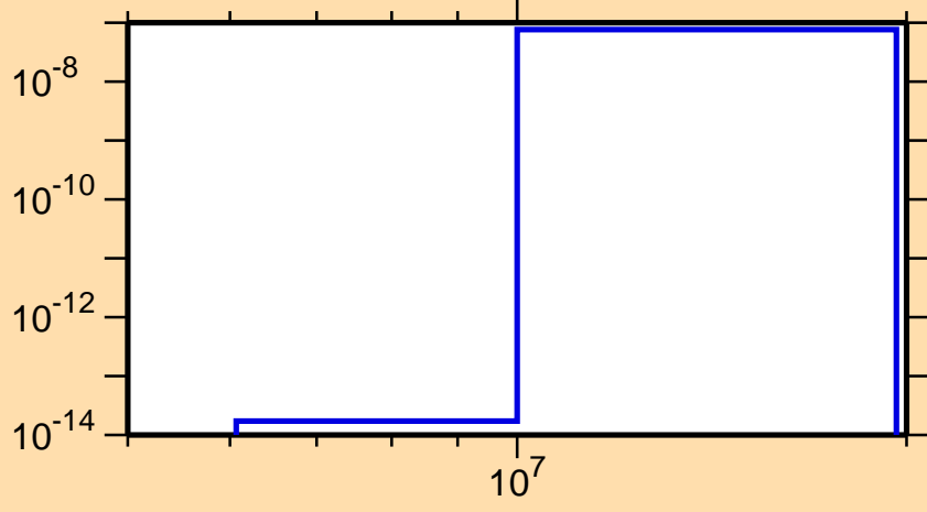
\sigma vs. E for ^{169}\text{Ta}(\text{mt } 45)
