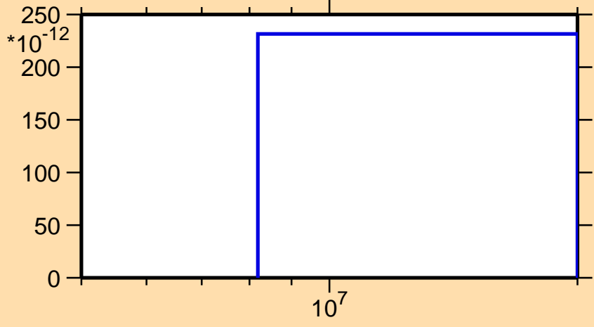
\sigma vs. E for ^{173}\text{Ta}(\text{mt } 45)
