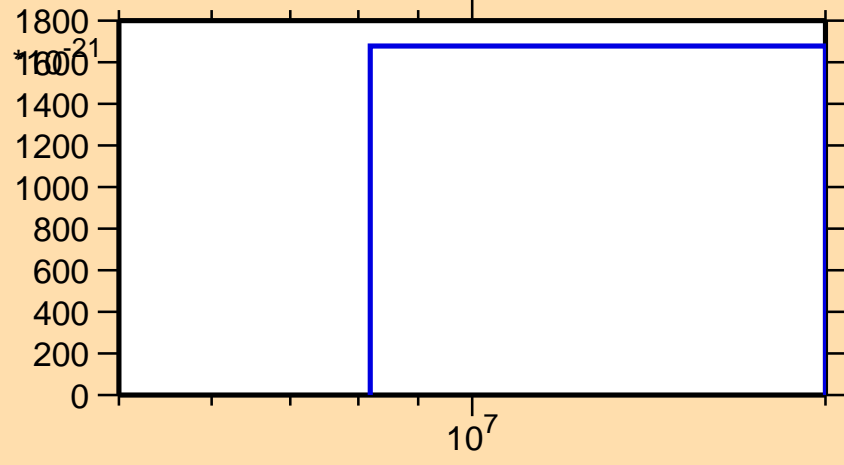
\sigma vs. E for ^{188}\text{Ta}(\text{mt } 42)
