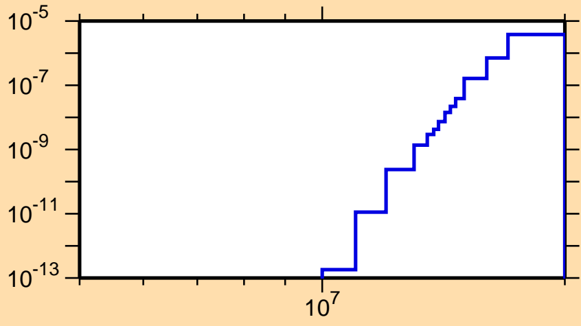
\sigma vs. E for ^{113}\text{Xe}(\text{mt } 34)
