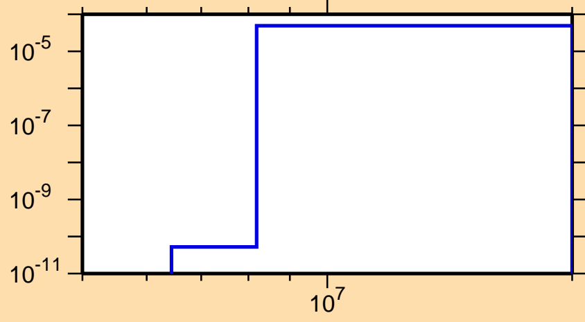
\sigma vs. E for ^{113}\text{Xe}(\text{mt } 45)
