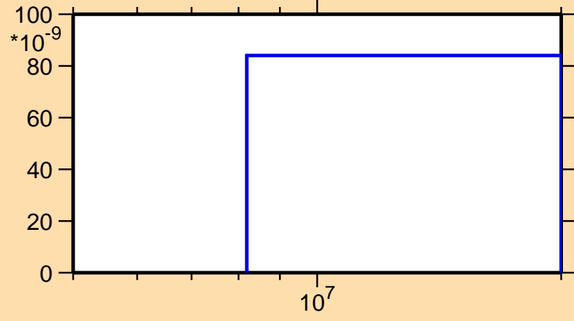
\sigma vs. E for ^{113}\text{Xe}(\text{mt } 34)
