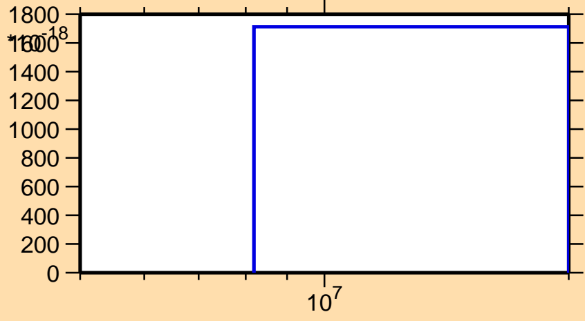
\sigma vs. E for ^{248}\text{Am}(\text{mt } 42)
