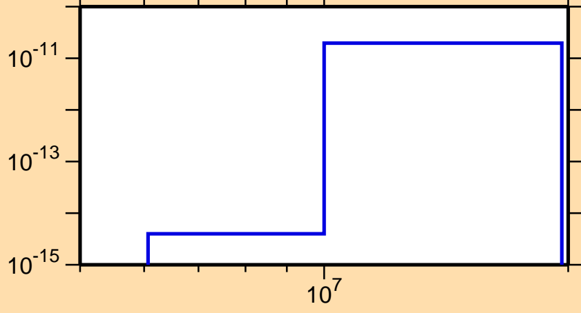
\sigma vs. E for ^{241}\text{Es} (mt 45)
