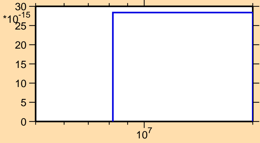
\sigma vs. E for ^{243}\text{Es} (mt 34)
