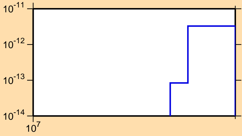
\sigma vs. E for ^{246}\text{Es} (mt 34)
