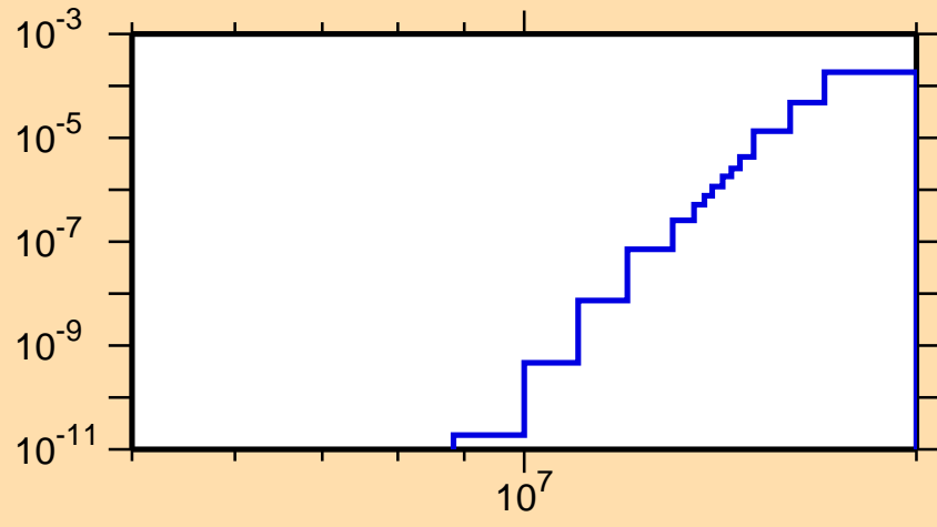
\sigma vs. E for ^{137}\text{Gd}(\text{mt } 45)
