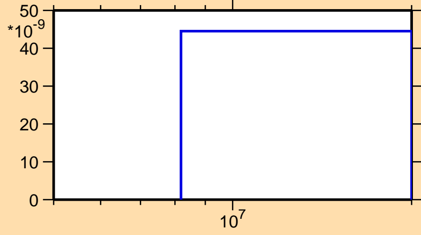
\sigma vs. E for ^{142}\text{Gd}(\text{mt } 45)
