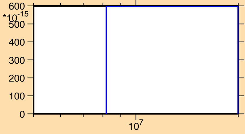
\sigma vs. E for ^{142}\text{Gd}(\text{mt } 34)
