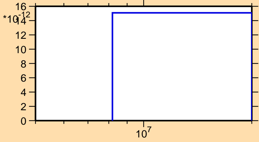
\sigma vs. E for ^{147}\text{Gd}(\text{mt } 45)
