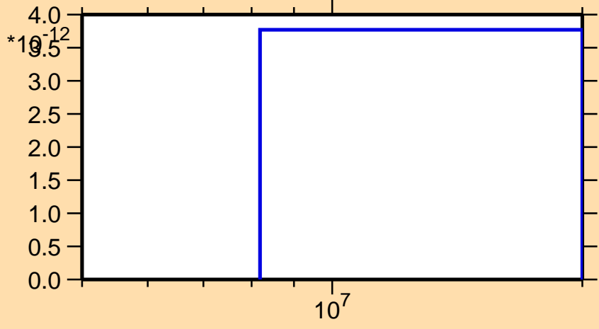
\sigma vs. E for ^{147}\text{Gd}(\text{mt } 34)
