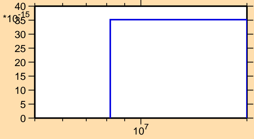
\sigma vs. E for ^{148}\text{Gd}(\text{mt } 34)
