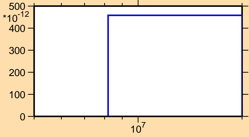
\sigma vs. E for ^{148}\text{Gd}(\text{mt } 45)
