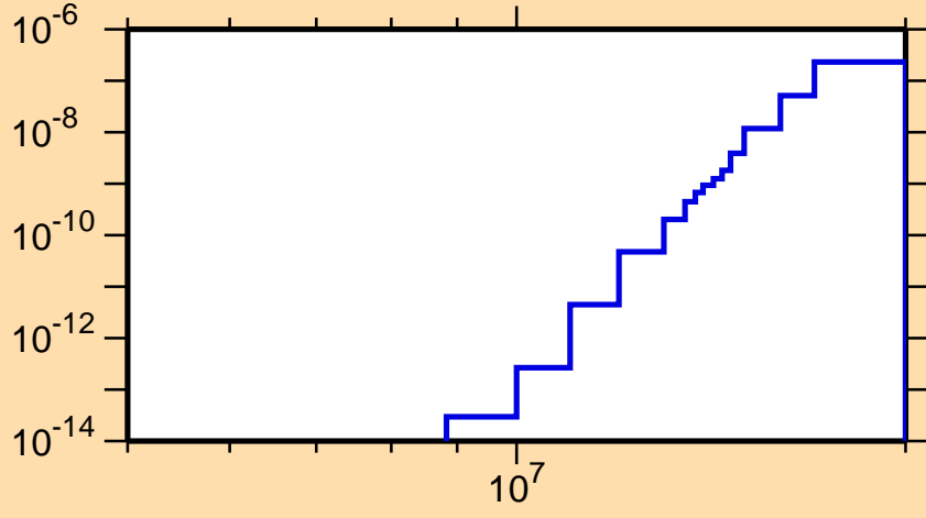
\sigma vs. E for ^{257}\text{Lw}(\text{mt } 45)
