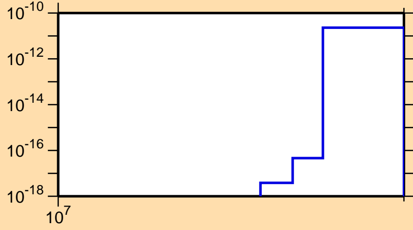
\sigma vs. E for ^{257}\text{Lw(mt 42)}
