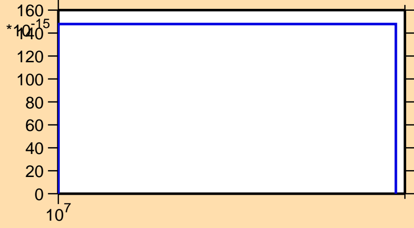
\sigma vs. E for ^{257}\text{Lw}(\text{mt } 42)
