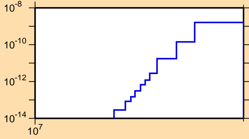
\sigma vs. E for ^{246}\text{Md}(\text{mt } 34)
