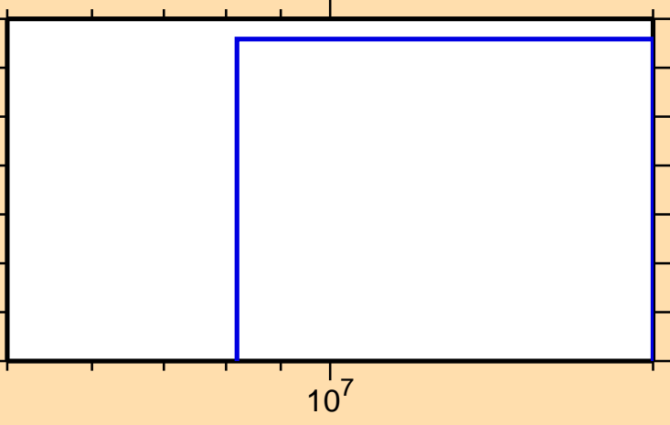
\sigma vs. E for ^{248}\text{Md}(\text{mt } 42)
