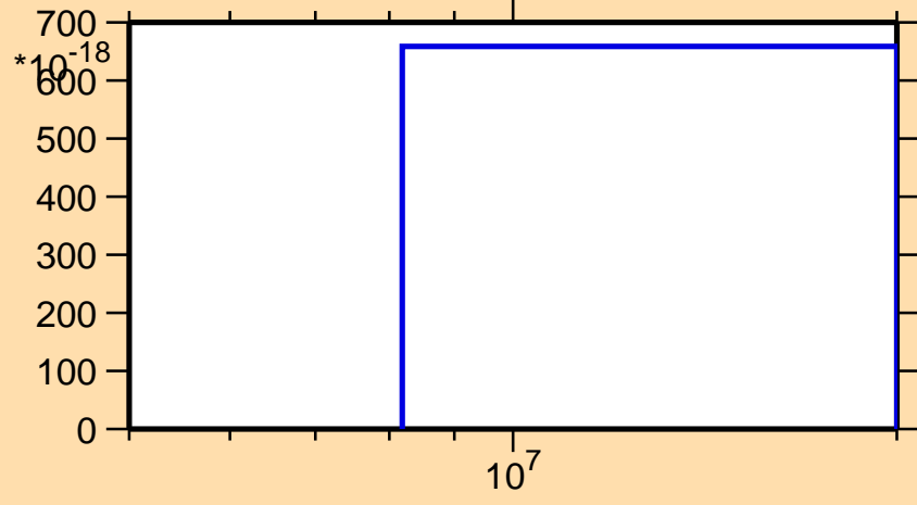
\sigma vs. E for ^{248}\text{Md}(\text{mt } 42)
