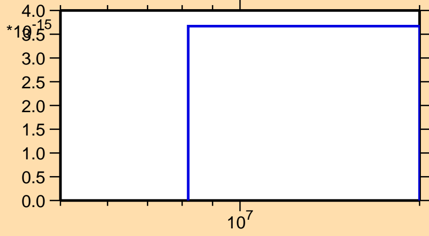
\sigma vs. E for ^{253}\text{Md}(\text{mt } 34)
