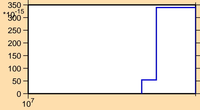
\sigma vs. E for ^{257}\text{No}(\text{mt } 45)
