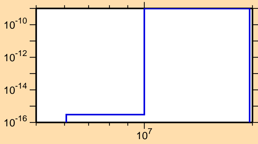
\sigma vs. E for ^{206}\text{At}(\text{mt } 45)
