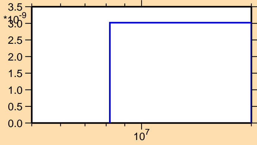
\sigma vs. E for ^{196}\text{Bi}(\text{mt } 45)
