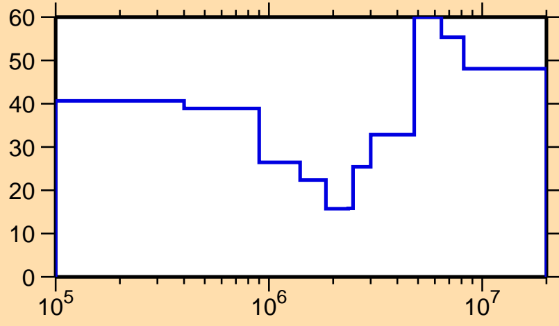
\Delta\sigma/\sigma vs. E for ^{173}\text{Dy}(n,incl.)
