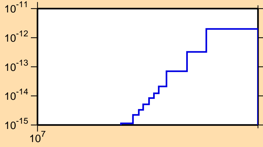
\sigma vs. E for ^{241}\text{Es} (mt 45)
