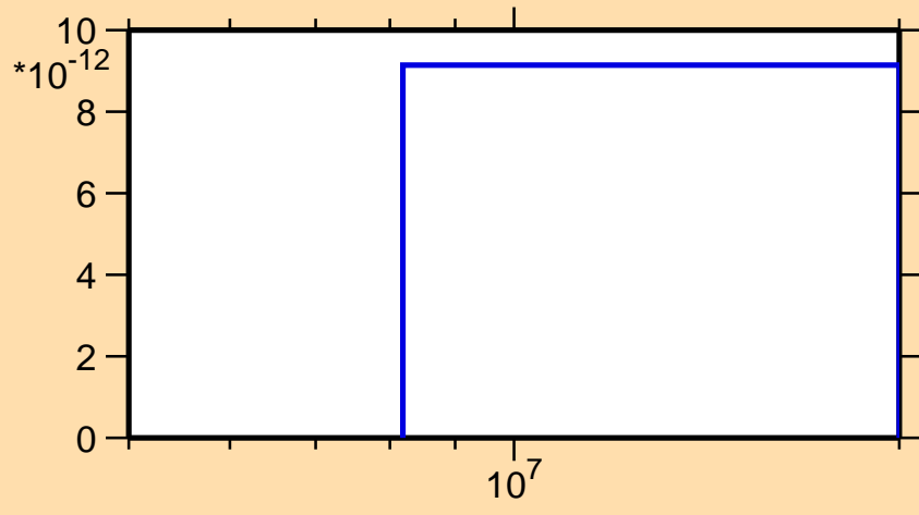
\sigma vs. E for ^{242}\text{Es} (mt 45)
