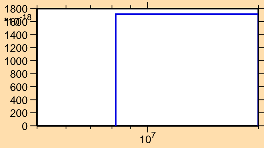
\sigma vs. E for ^{248}\text{Es} (mt 34)
