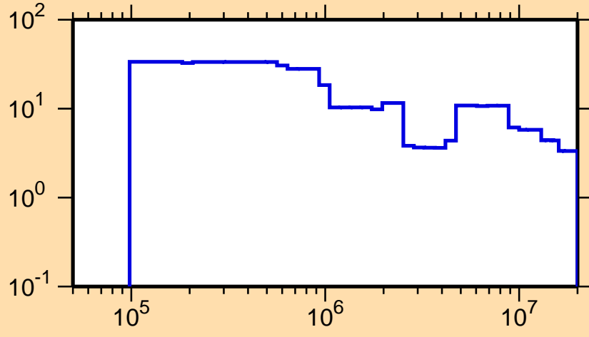
\Delta\sigma/\sigma vs. E for ^{257}\text{Fm}(n,tot.)
