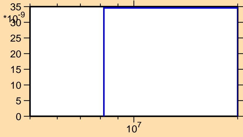
\sigma vs. E for ^{206}\text{Fr}(\text{mt } 45)
