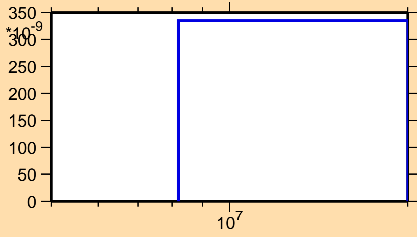
\sigma vs. E for ^{66}\text{Ga} (mt 45)
