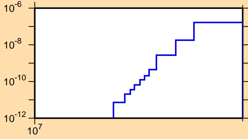
\sigma vs. E for ^{139}\text{Gd}(\text{mt } 34)
