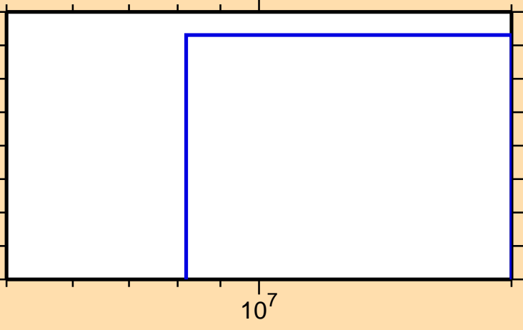
\sigma vs. E for ^{148}\text{Gd}(\text{mt } 34)
