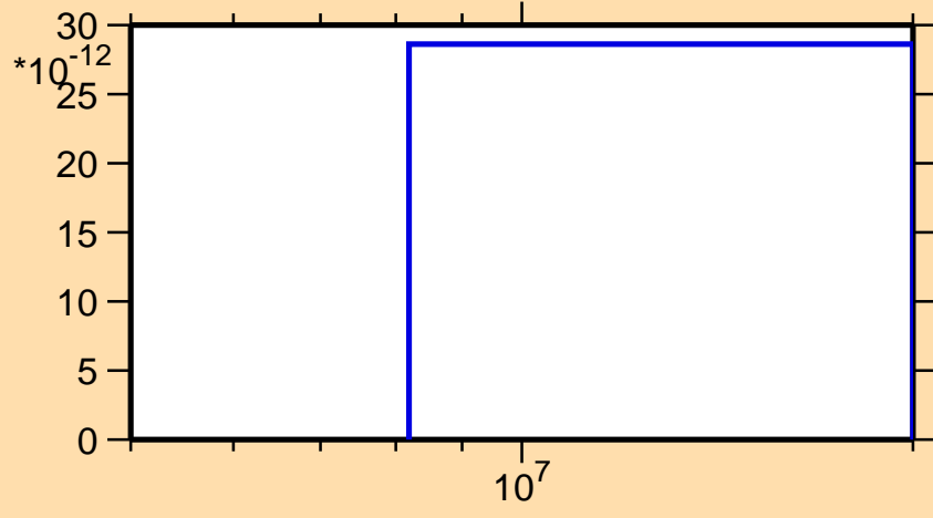
\sigma vs. E for ^{64}\text{Ge}(\text{mt } 34)
