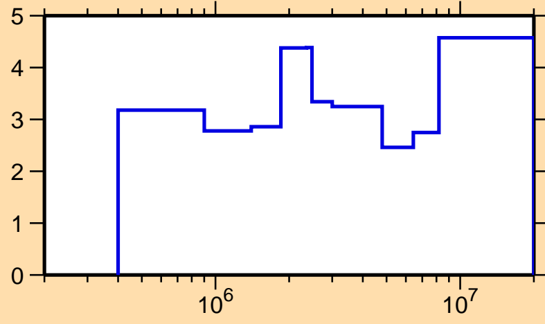
\Delta\sigma/\sigma vs. E for ^{73}\text{Ge}(n,el.)
