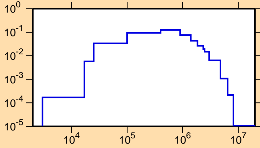
\sigma vs. E for ^{73}\text{Ge}(n,n_1)
