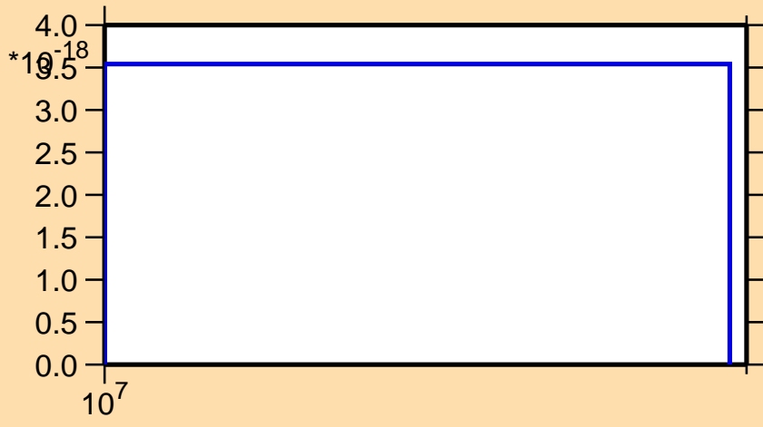
\sigma vs. E for ^{76}\text{Ge}(n,nt)
