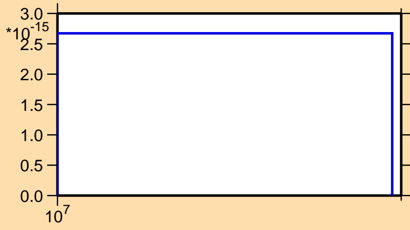
\sigma vs. E for ^{77}\text{Ge}(n,nt)
