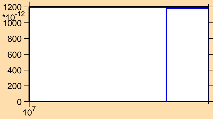
\sigma vs. E for ^{81}\text{Ge}(n,nt)
