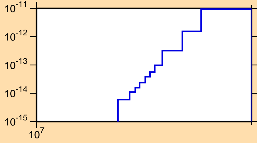
\sigma vs. E for ^{254}\text{Lw}(\text{mt } 45)
